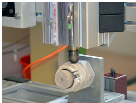
Schlagprüfung / Impact resistance
