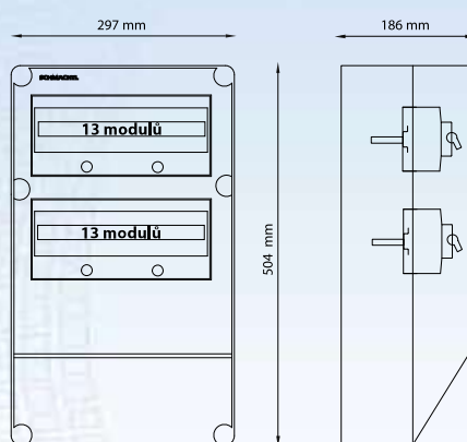
SKŘÍŇ S 26M
