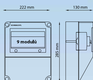
SKŘÍŇ S 9M
