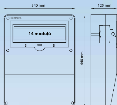
SKŘÍŇ S 14M
