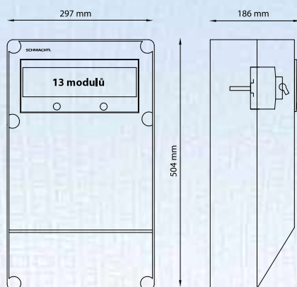
SKŘÍŇ S 13M
